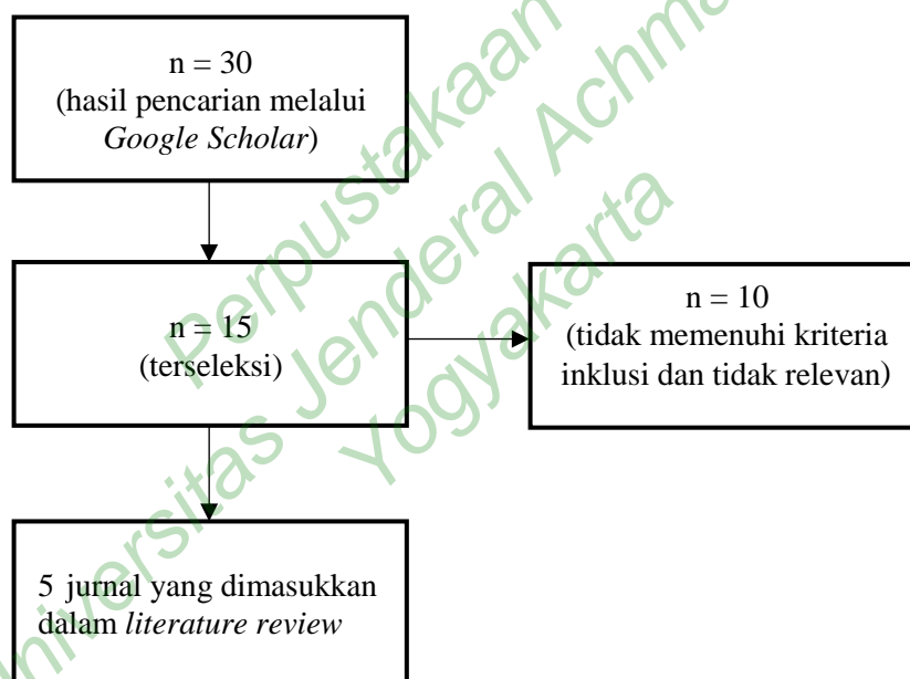
Gambar 2.1 seleksi studi
