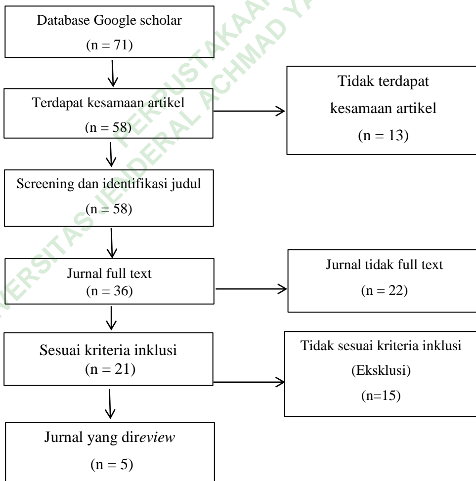
Gambar 3.1 Seleksi Studi
