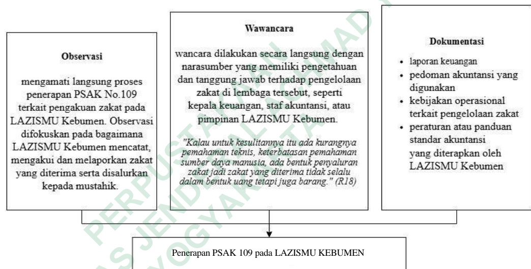
Gambar 4. 1 Kerangka Berpikir
